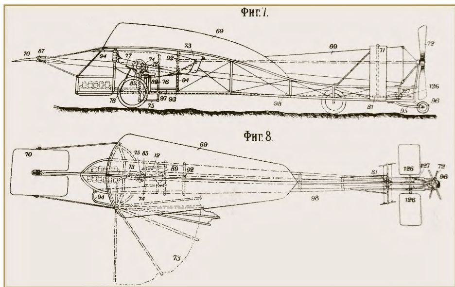
Чертеж аэроплана конструкции полковника С. Люпова
