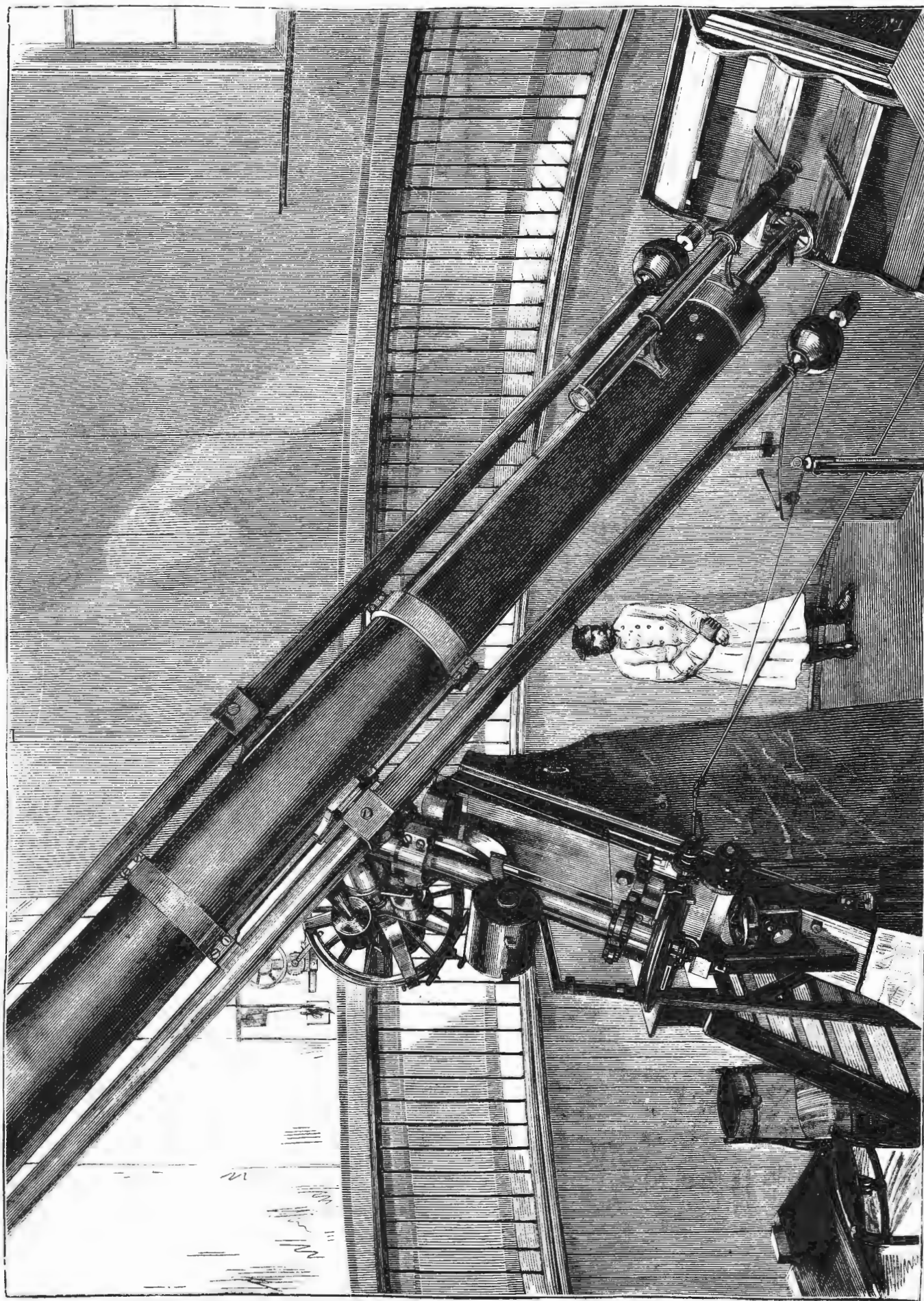
Николаевская Главная Астрономическая Обсерваторія въ Пулковѣ. Большой Рефракторъ для изслѣдованія двойныхъ звездъ. Рис. Подольскій, грав. Кононжевскій.
