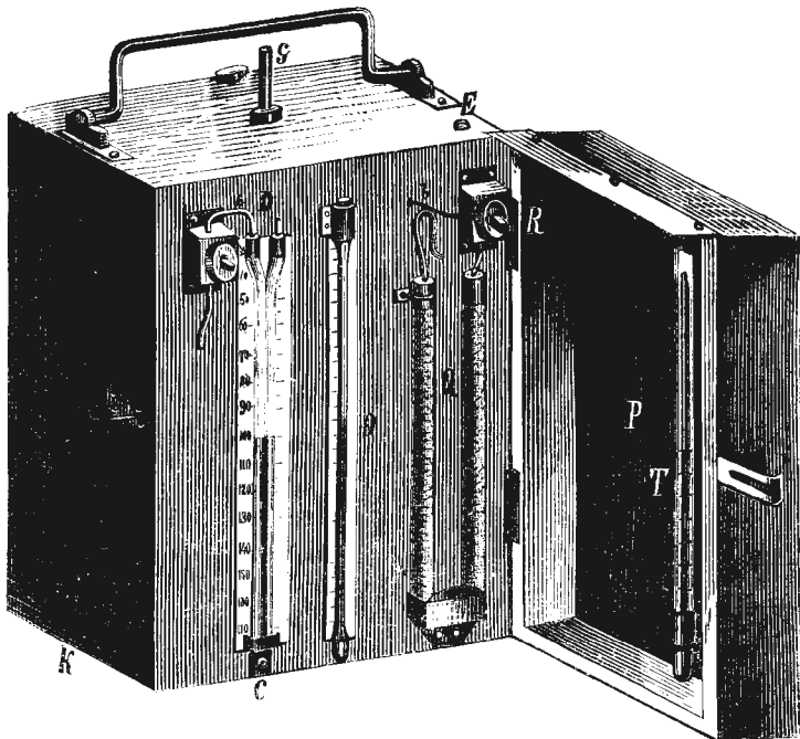
Высотомѣръ Проф. СПб. Унив. Д. И. Менделѣева.
