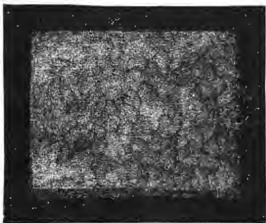
Поверхность солнца. Общій видъ.
