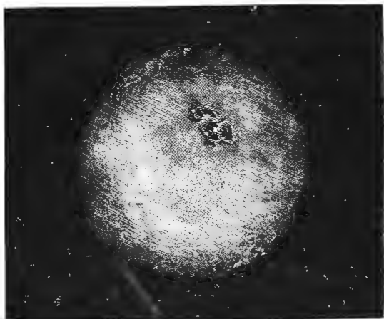
Фотографическій снимокъ съ солнца.
