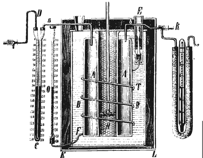
Высотомѣръ Проф. СПб. Унив. Д. И. Менделѣева.
