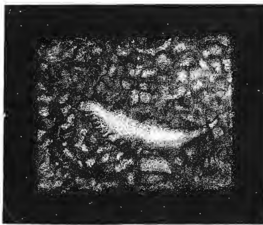
Рисовыя зерна и свѣлое пятно.
