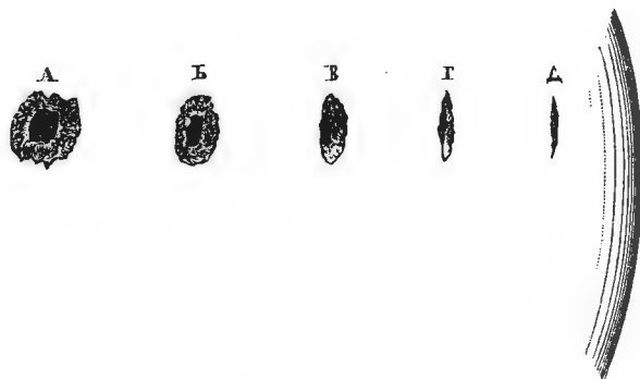
Наглядное представленіе перемѣщенія солнечнаго пятна.
