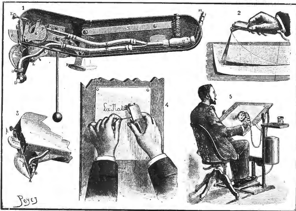
Воздушная кисть. 1) Внутреннее расположеніе механизма. 2) Дѣйствіе кисти. 3) Конечность кисти. 4) Воспроизведеніе тонкихъ штриховъ. 5) Общій видъ аппарата. По рис. Н., грав. Пойэ.
