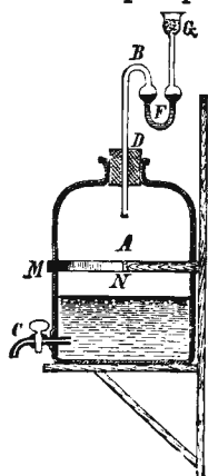
Чертежъ прибора для храненія кипяченой воды.
