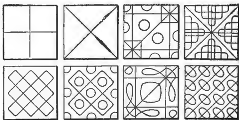
Рис. 12. Хладниевы фигуры.
