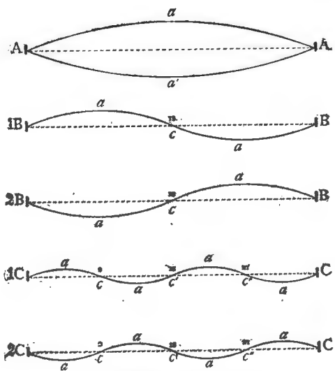
Рис. 10. Колебанія струны.
