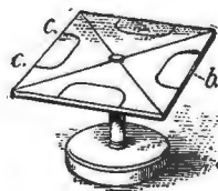
Рис. 11. Хладниева пластинка.
