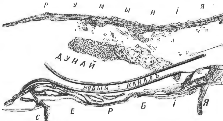
Исправленіе дунайскаго русла у „Желѣзныхъ Воротъ“. Новый каналъ.
