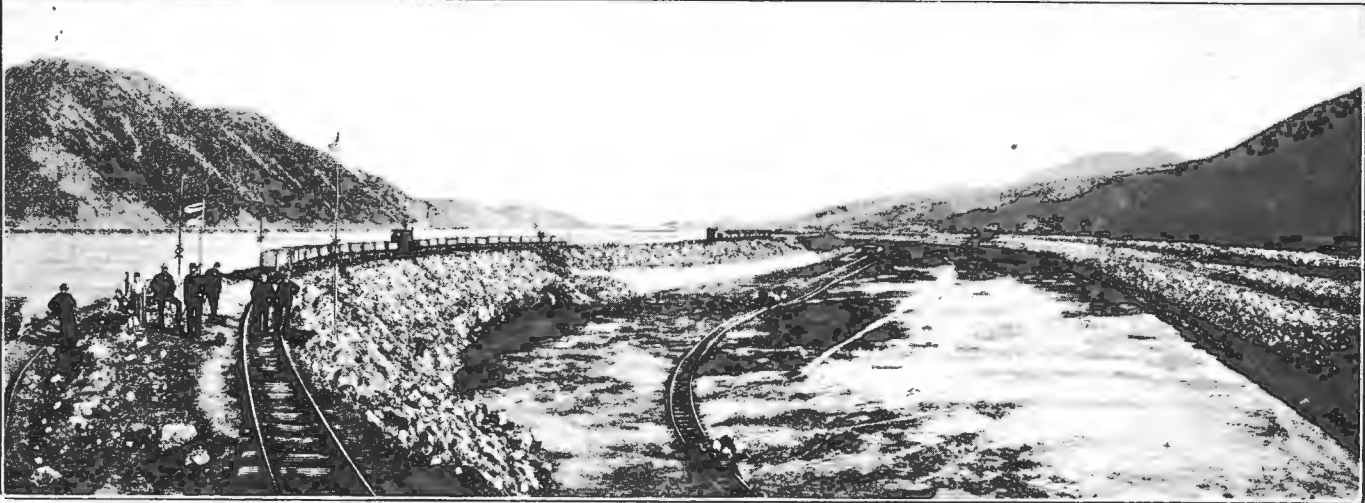
Исправленіе дунайскаго русла у „Желѣзныхъ Воротъ“. Видъ судоходнаго канала.
