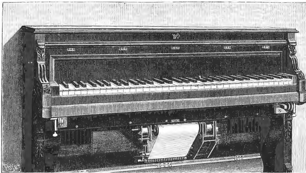
Приборъ, записывающій музыку. — Рис. 3. Наружный видъ прибора.
