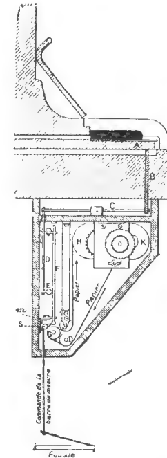
Приоръ, записывающій музыку. — Рис. 2. Внутренний видъ въ продольномъ разрѣзѣ.
