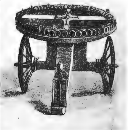
Круглая батарея времени полтавскаго боя. (С.-Петербургскій Артиллерійскій музей).
