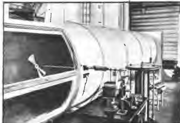
Труба с электрическим вентилятором для производства изысканий надъ сопротивлением воздуха и работою различных родов винтов.
