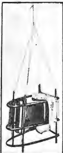
Метеорологическая переносная станция с самозаписывающими приборами.
