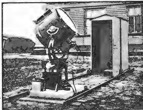
Электрический прожектор для ночного наблюдения за воздушными течениями по облакам.
