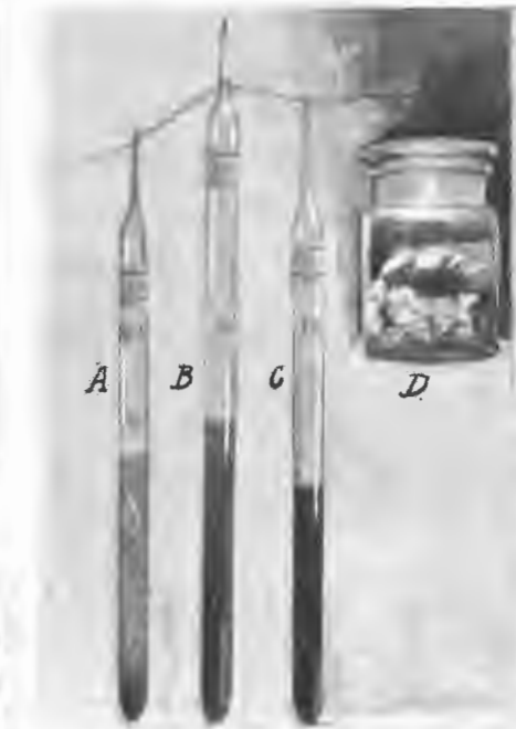
Превращение изопрена в каучук. А—запаянный сосуд с изопреном; стрелкой обозначен кусочек введенного металлического натрия. На дубь начинает оседать искусственный каучук (на 2-й день). В—то же на 3-й день. С—на 4-й день весь изопрен превратился в каучук. Д—сосуд с кусками искусственного каучука.
