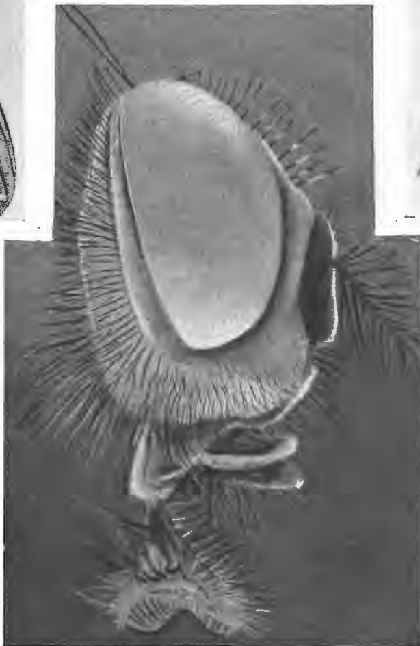
Рис. 4. Глазъ муhy, — видъ сбоку при сильномъ увеличеніи.
