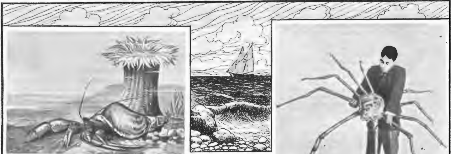
Сожительство рака-отшельника и актинии.
