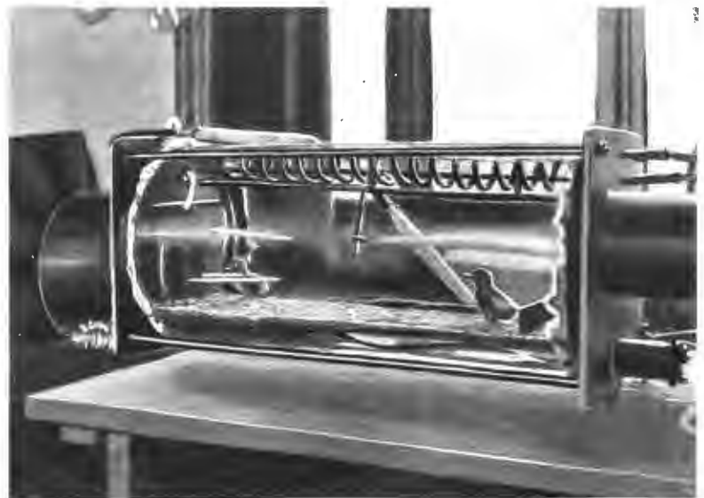
Рис. 3. Выведенные въ безмикробномъ аппаратѣ цыплята.
