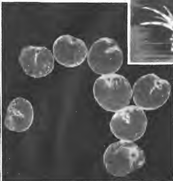
Животное, причиняющее свечение моря— Noctiluca millaris .
