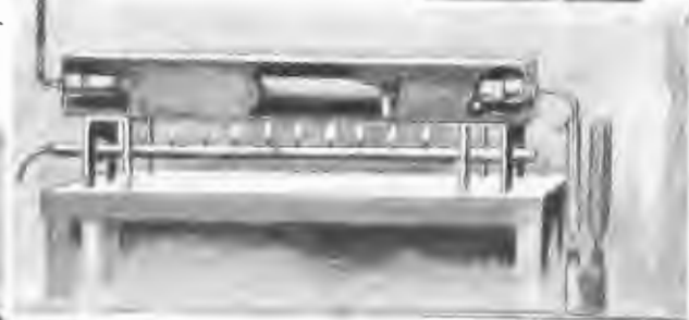
Тот же прибор в разрезе. Железные трубки, содержащее вещество, поглощающее соляную кислоту, нагреваются газовой горелкой. Дихлорит наливается в воронку. Изопрен, охлаждаясь, поступает в сосуд.
