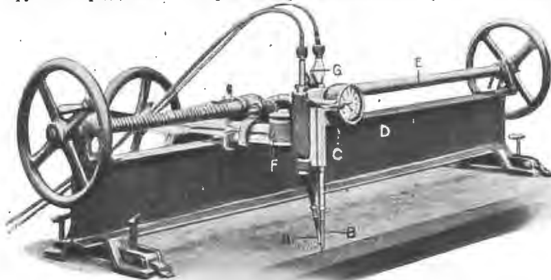
Рис. 2. Снарядъ для разрѣзанія, посредствомъ пережиганія, желѣзныхъ пластинъ.
