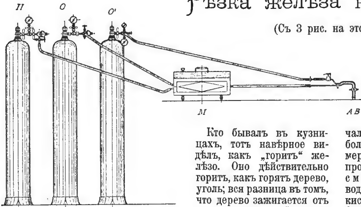
Рис. 1. Схематический рисунокъ, представляющій устройство для пережиганія желѣза кислородомъ.
