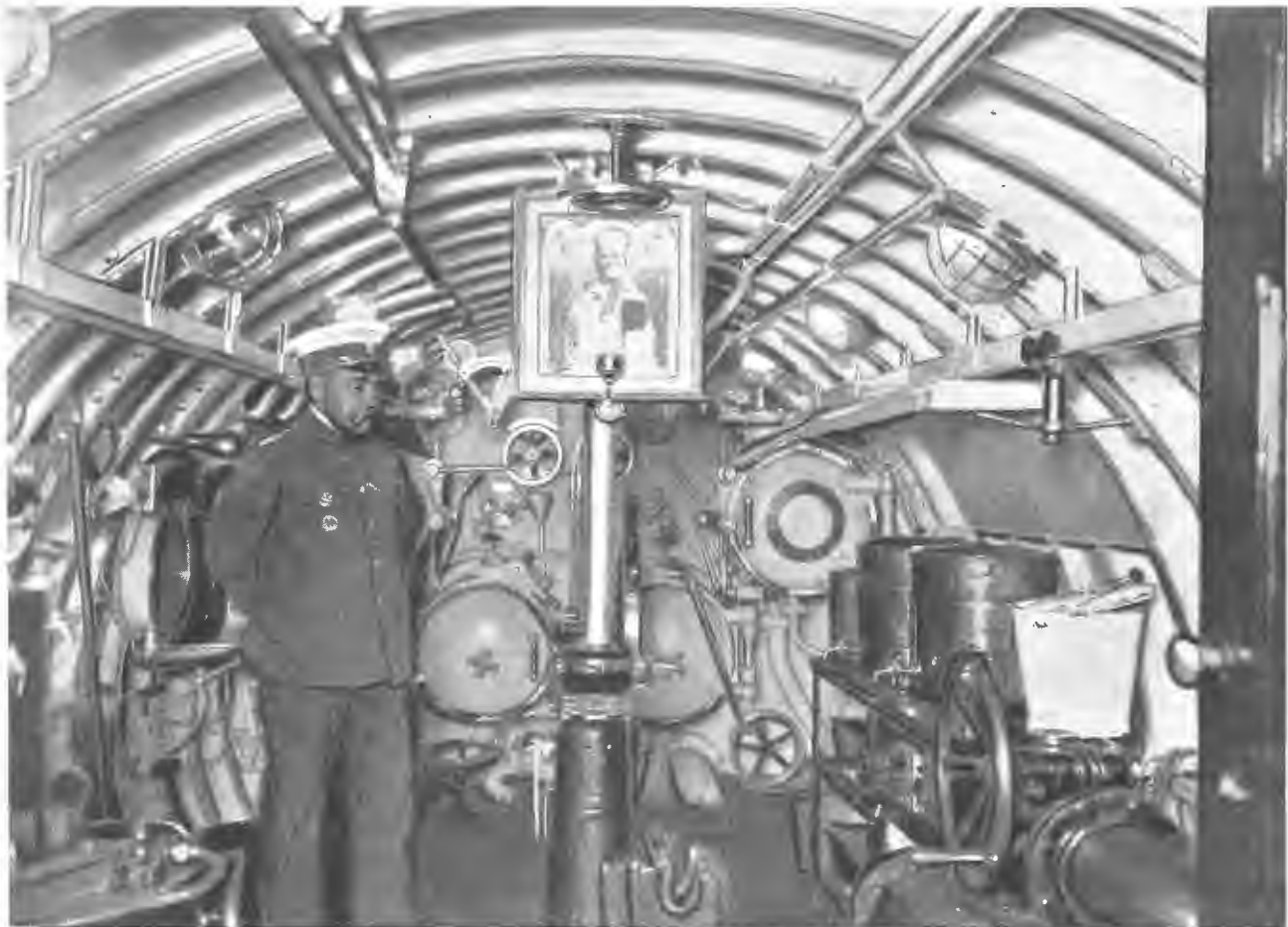
Внутренность носовой части подводной лодки. Направо—электрическая кухня.
