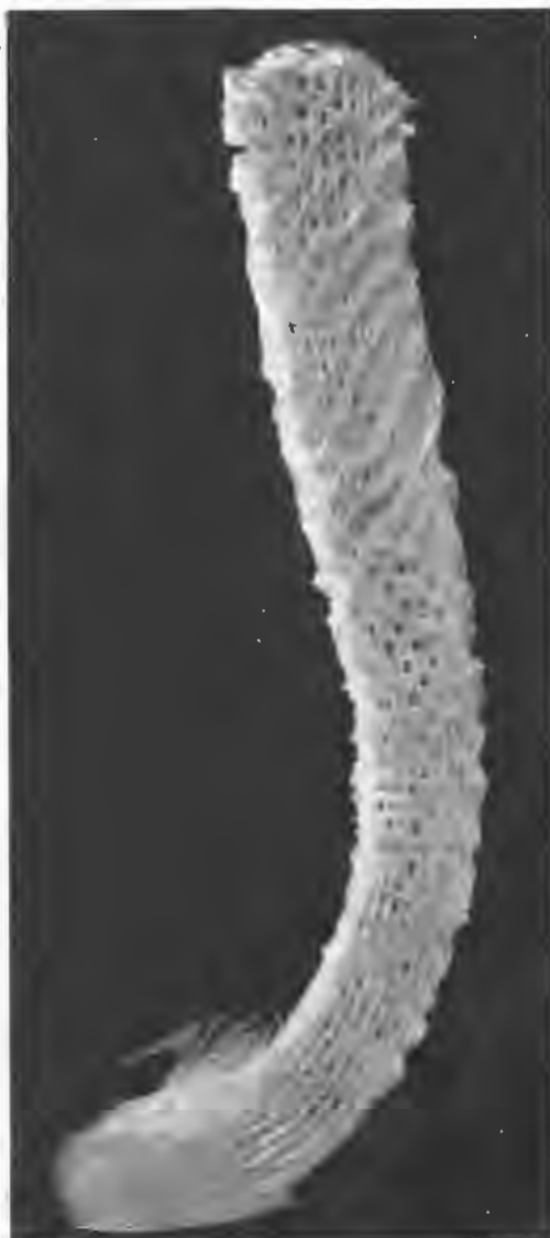
Стекловидная губка Euplectella aspergillum .
