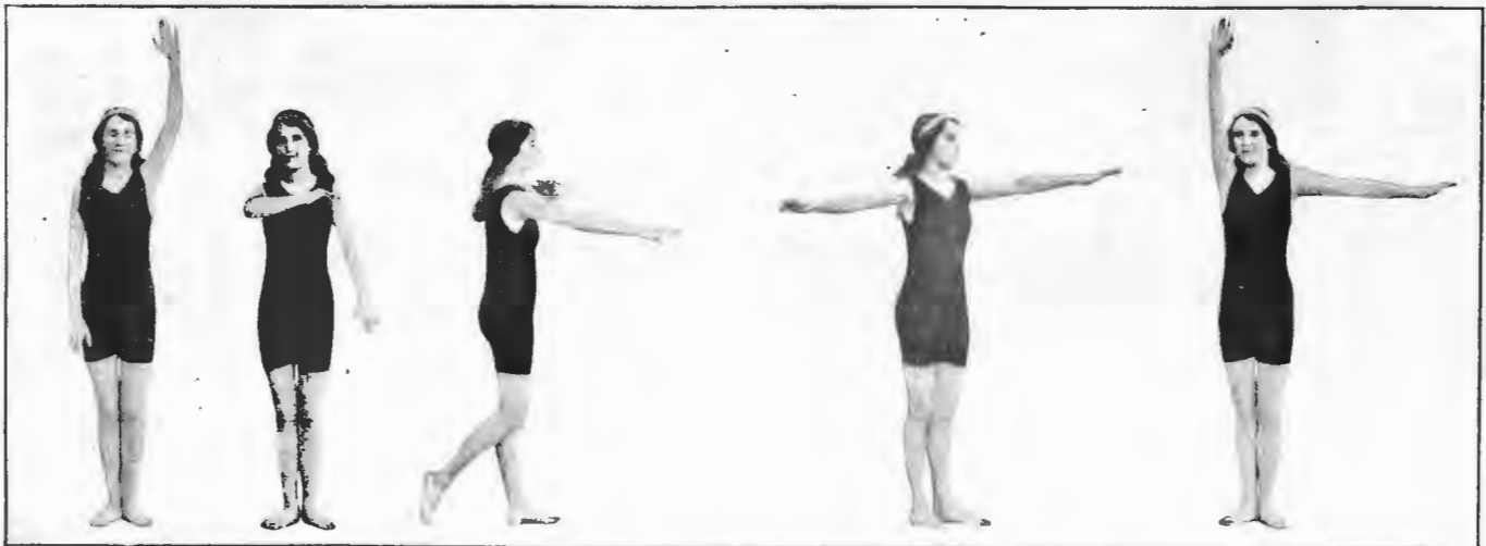
Школа ритмической гимнастики Жака Далькроза въ Хеллерау (близъ Дрездена). Упражненія. Пластическій канонъ въ 5/4.
