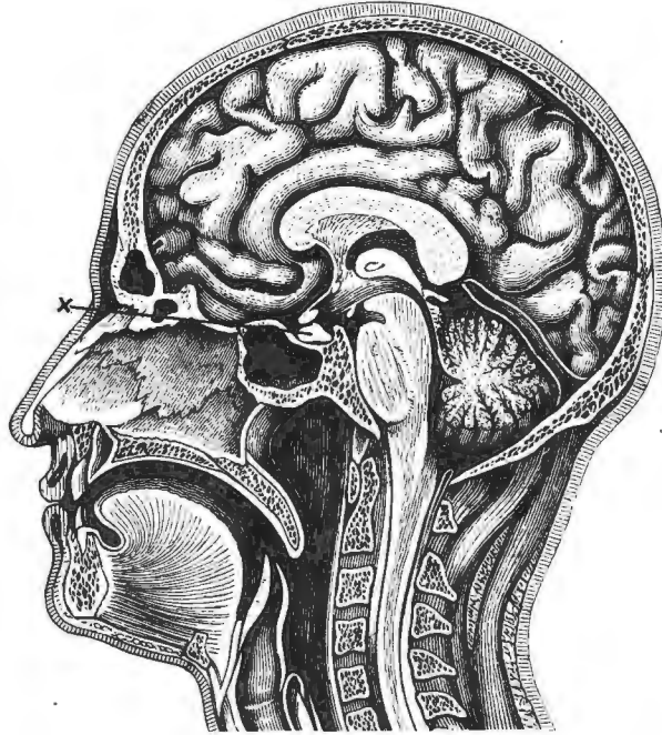
× Мозговой придатокъ. Рис. 1. Поперечный разрѣзъ мозга.
