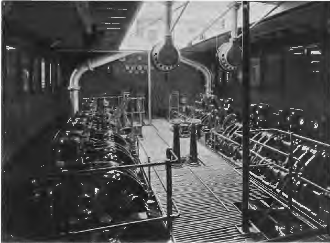
„Теплоходы“. Машинное отделение на теплоход „Бородино“. Дизель-моторы.
