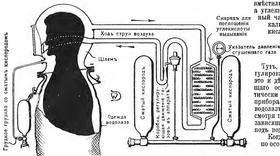
1. Схема устройства безтрубчатого аппарата для снабжения водолаза воздухом.
