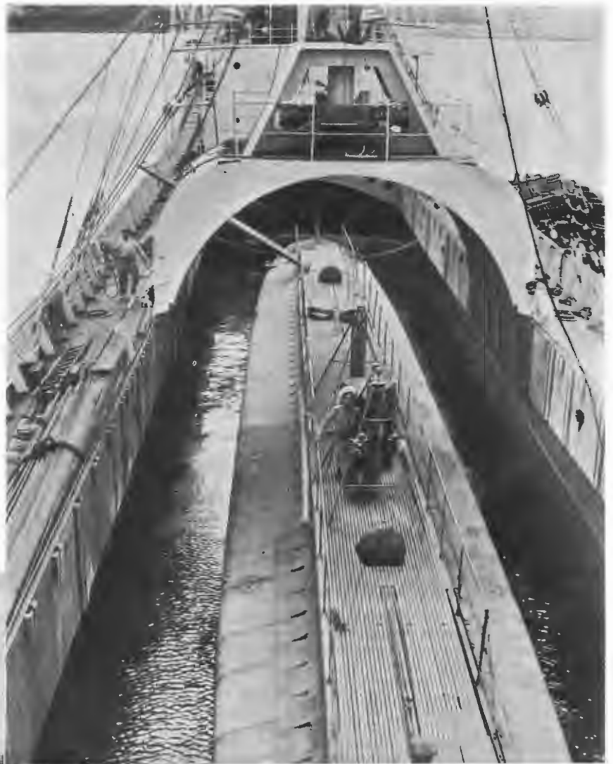
Подводная лодка въ полномъ снаряженiи съ командой внутри транспорта „Кенгуру“.
