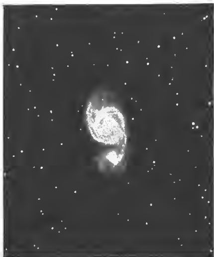
Рис. 4. Спиральная туманность въ созвѣздіи Гонимыхъ Псовъ.
