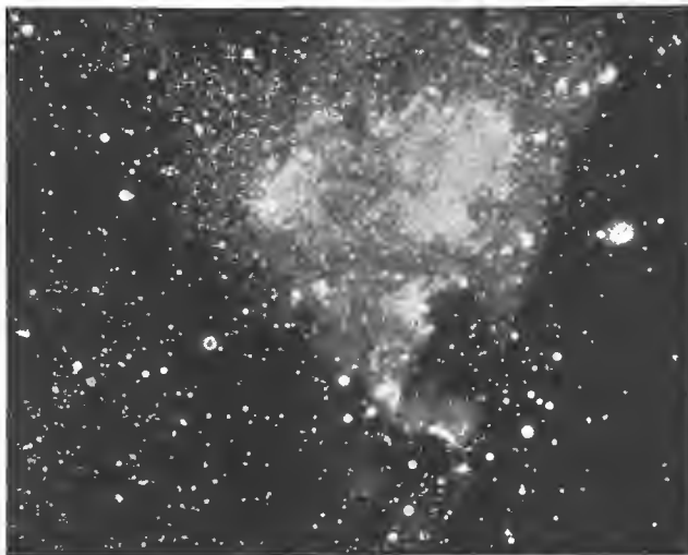
Рис. 3. «Американская» туманность въ созвѣздіи Лебеда.
