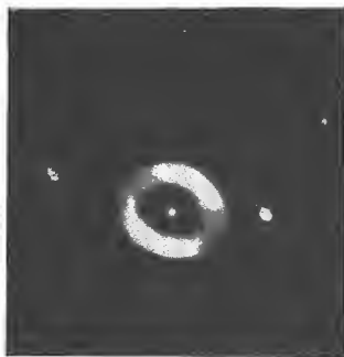
Рис. 6. Кольцеобразная туманность в созвездии Лиры.
