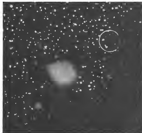
Рис. 12. Новая Звѣзда Персея, по снимку, сдѣланному спустя 54 дня.
