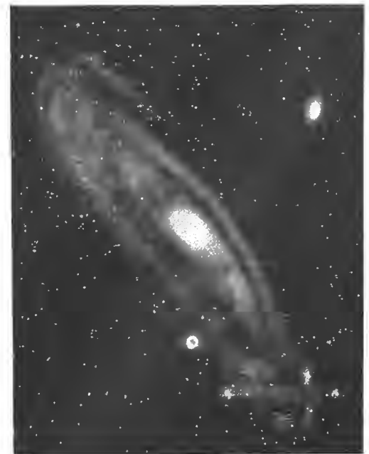
Рис. 5. Большая туманность въ созвѣздіи Андромеды.
