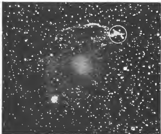
Рис. 11. Новая Звѣзда Персея, по снимку 20 сентября 1901 г.
