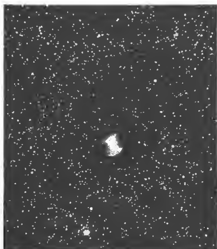
Рис. 9. Туманность в созвездии Лисички.
