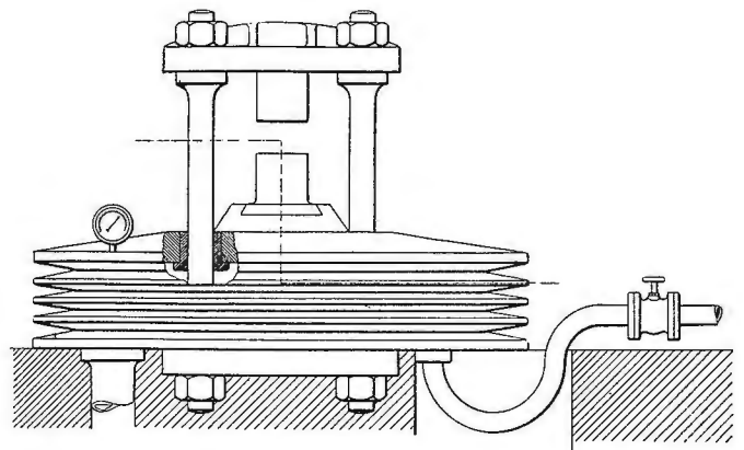
Схема гидравлическаго пресса Татаринова.
