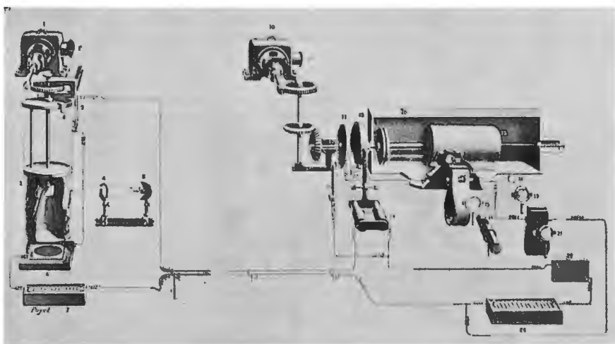
Станція отправленія: 1) Двигатель. 1а) Счетчикъ оборотовъ двигателя. 2) Стеклянный цилиндръ, на который накладывается негативъ на пленкѣ. Наружный металлическій кожухъ на этомъ цилиндрѣ на рис. не представленъ. 3) Лампа. 4) Чечевица-конденсаторъ свѣта, идущаго отъ лампы. 5) Призма, направляющая свѣтъ на селень. 6) Селеновая пластинка. 7) Электрическая батарея. 8, 9) Приспособленія для установокъ одновременности вращенія цилиндровъ на обѣихъ станціяхъ. Приемная станція: 10) Двигатель. 11, 12) Приспособленія для установокъ одновременности хода цилиндровъ. 13) Приемный цилиндръ, на который наложена фотографическая пленка, для запечатлѣнія передаемаго изображенія. 14) Лампа. 15) Конденсаторъ свѣта. 16) Гальванометръ, для регулированія силы свѣта и введенія его въ точное соответствіе съ тѣмъ, какой отправленъ съ первой станціи. 17) Чечевица, черезъ которую впускается свѣтъ въ цилиндръ, на фотографическую пленку. 18 по 22) Части конденсатора, снаряда для уравненія дѣйствія селена (именно: 18) лампа, 19) чечевица-конденсаторъ, 20) гальванометръ, 21) конденсаторъ и 22) пластинка селена). 23) Электрическая батарея. 24, 25) Части приспособленія для установокъ одновременности движенія цилиндровъ. 26) Кожухъ надъ цилиндромъ съ пленкою. 27 и 28) Части приспособленія для уравненія времени вращенія цилиндровъ.
